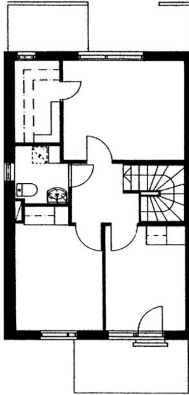
Kurkijointie 5 G 25 / pohjakuva 2.kerros Ei mittakaavassa
