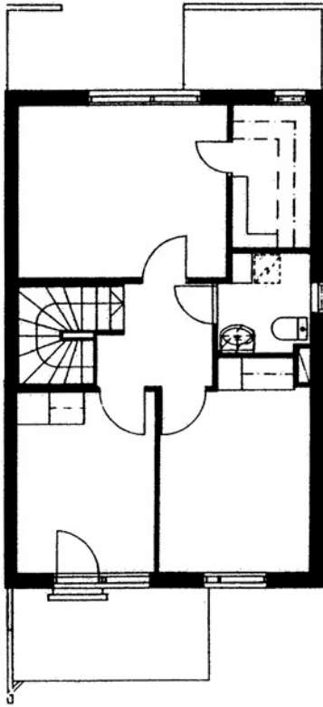
Kurkijointie 5 B 5 / pohjakuva 2.kerros Ei mittakaavassa
