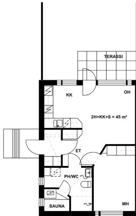
Suhosenmutka 1 A 1 / Pohjakuva Ei mittakaavassa
