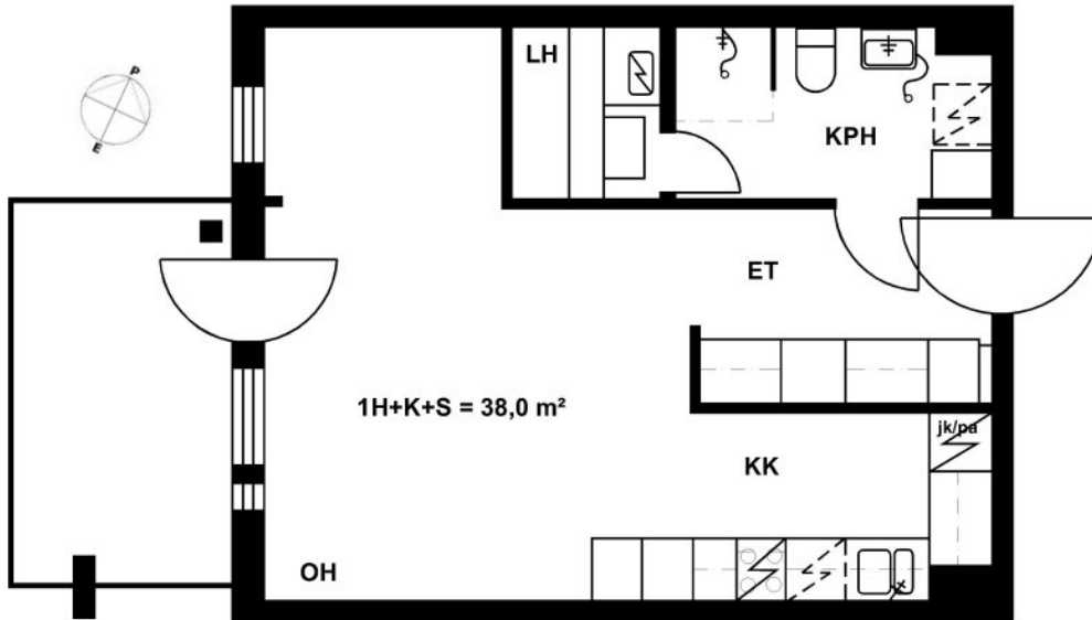
Pikisaarencatu 41 A 4 / Pohjakuva Ei mittakaavassa
