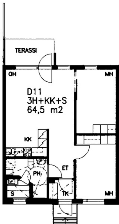
Juvanpuisto 1 D 11 / pohjakuva Ei mittakaavassa
