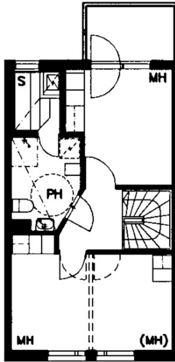
Juvanpuisto 1 B 4 / pohjakuva 2.kerros Ei mittakaavassa
