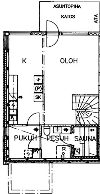
Taavinharju 16 E 10 / pohjakuva 1.kerros Ei mittakaavassa
