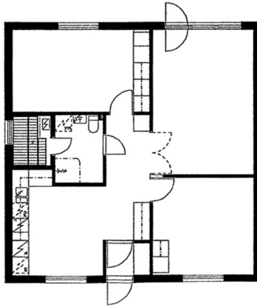
Trappukorventie 2 C 9 / pohjakuva Ei mittakaavassa
