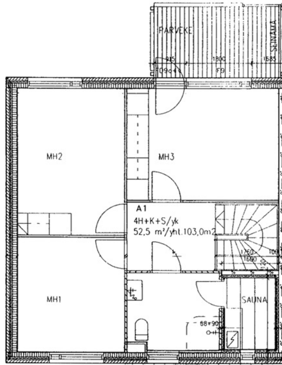
Rauduntie 12 E 9 / pohjakuva 2. kerros Ei mittakaavassa
