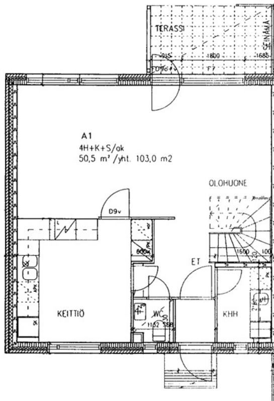
Rautuntie 12 E 9 / pohjakuva 1. kerros Ei mittakaavassa
