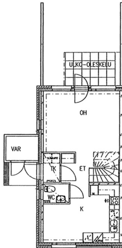
Santakuopankuja 11 C 11 / pohjakuva 1. kerros Ei mittakaavassa
