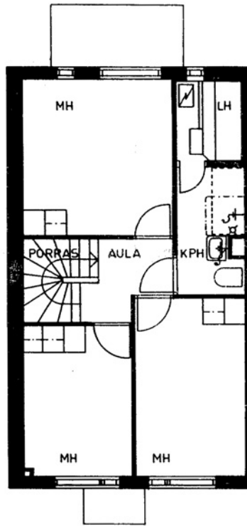
Jpuankatu 24 D 20 / pohjakuva 2.kerros Ei mittakaavassa
