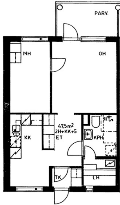
Jepuankatu 24 E 26 / pohjakuva Ei mittakaavassa
