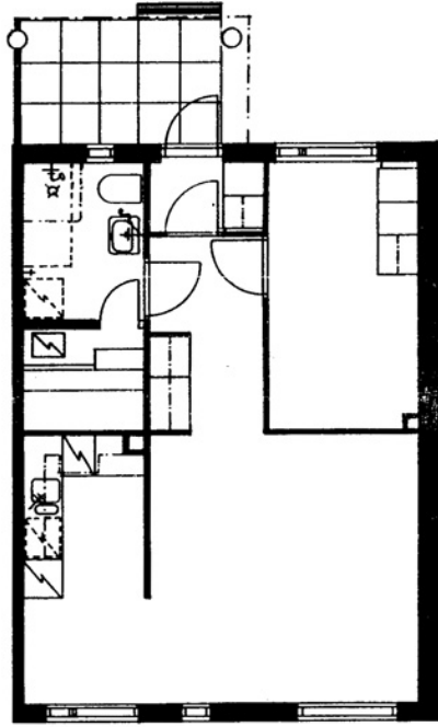
Jepuankatu 24 E 24 / pohjakuva Ei mittakaavassa
