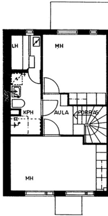
Jepsänkät 24 H 45 / pohjakuva 2.kerros Ei mittakaavassa
