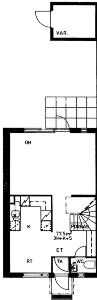
Jpuankatu 24 H 45 / pohjakuva 1.kerros Ei mittakaavassa
