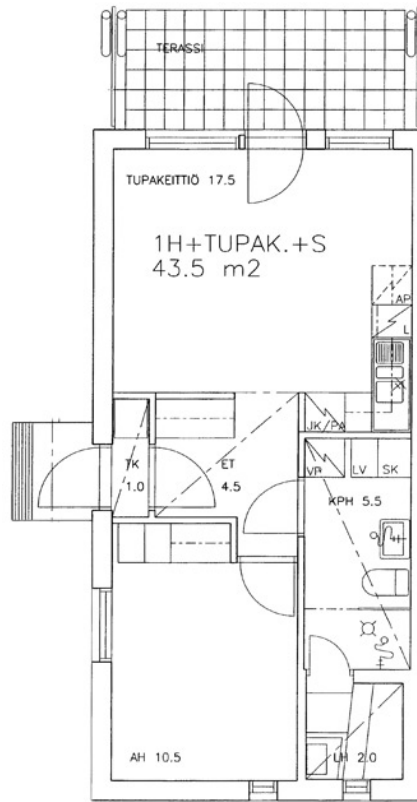
Esterinkatu 39 B 5 / pohjakuva Ei mittakaavassa
