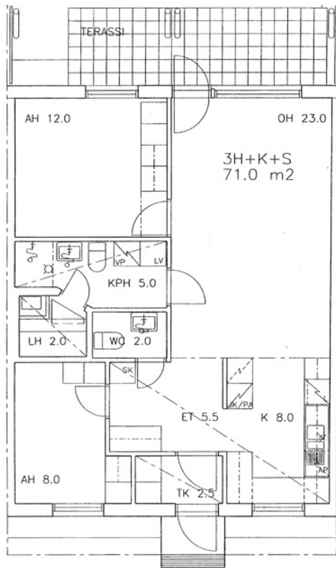
Esterinkatu 39 A 4 / pohjakuva Ei mittakaavassa
