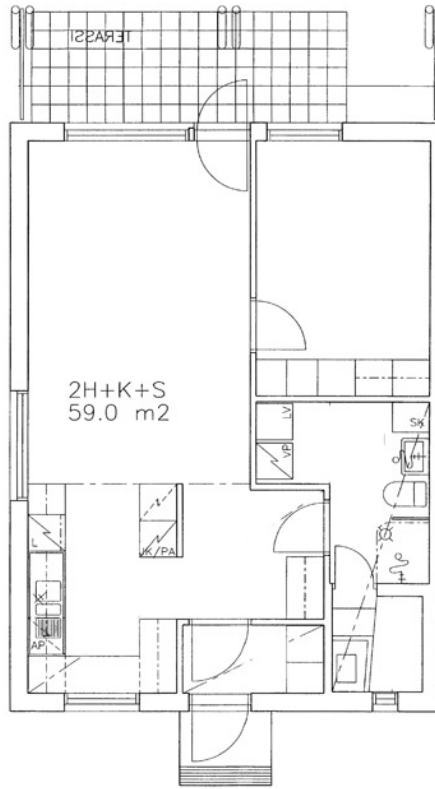
Esterinkatu 39 C 12 / pohjakuva Ei mittakaavassa
