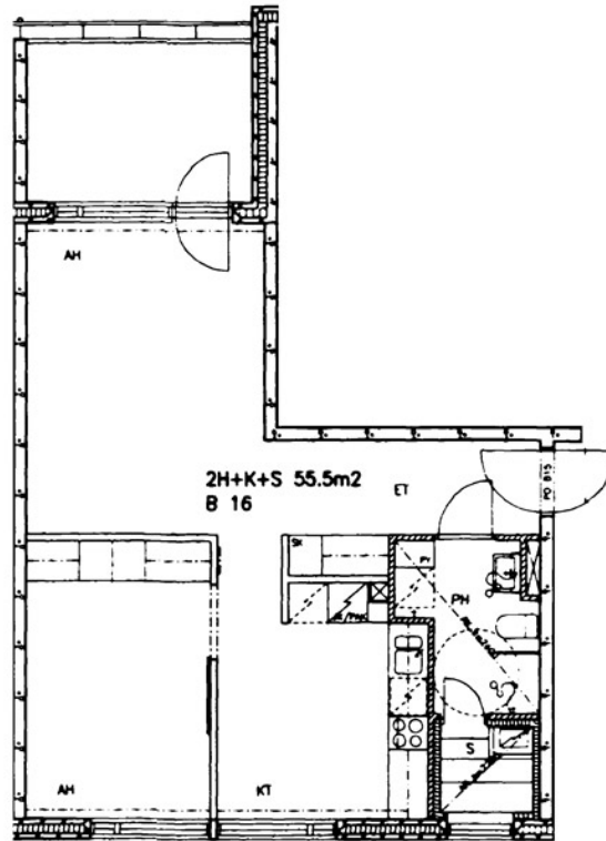
Paciuksenkaari 6 B 28 / pohjakuva Ei mittakaavassa
