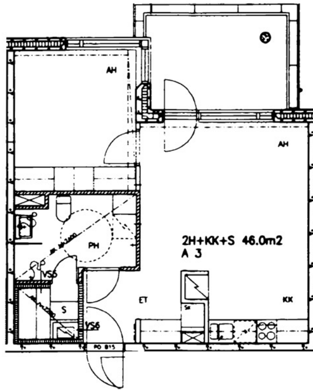
Paciuksenkaari 6 A 7 / pohjakuva Ei mittakaavassa
