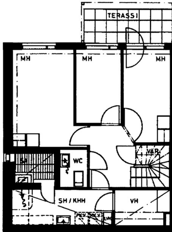
Nousutie 18 A1 / pohjakuva 1. kerros Ei mittakaavassa
