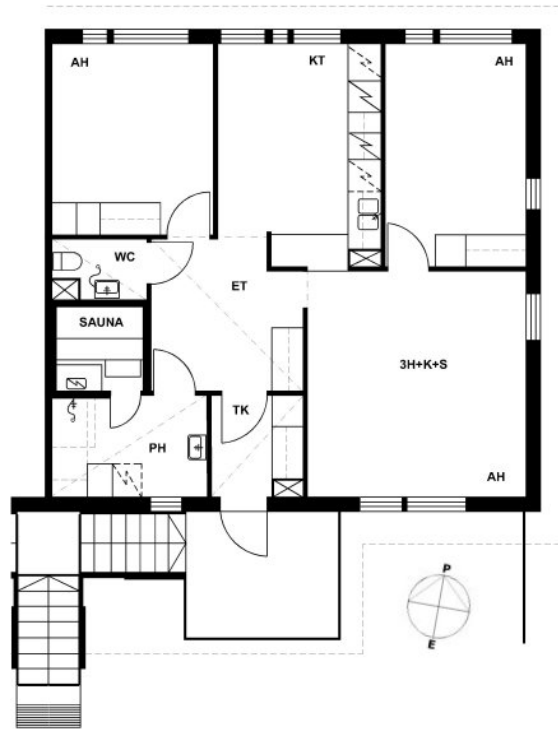
Kotikaivonpolku 2 A 4 / Pohjakuva Ei mittakaavassa
