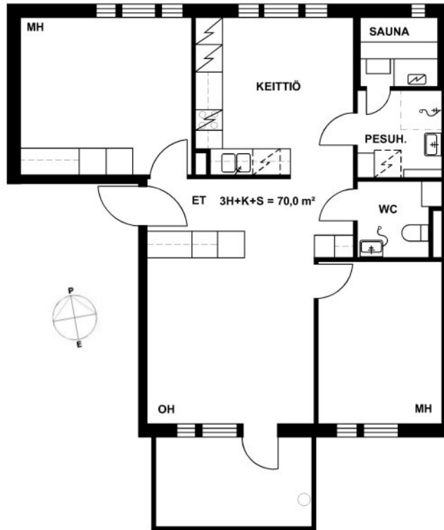
Moisionkuja 1 B 14 / Pohjapiirustus Ei mittakaavassa
