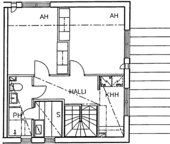
Tikkurikuja 10-12 B 2 / pohjakuva 2. kerros Ei mittakaavassa
