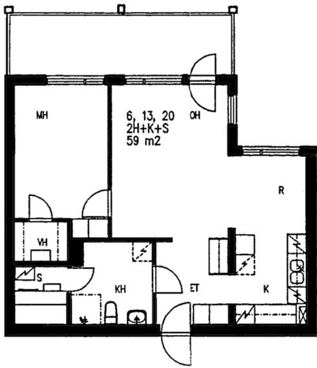
Pähkinämäentie 231 As 6 / Pohjakuva Not in scale
