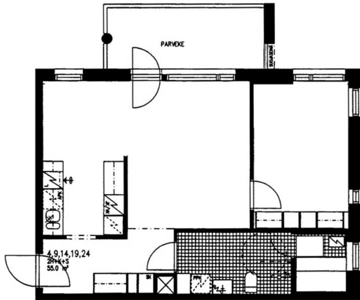
Särkilahdenkatu 1 A 14 / pohjakuva Ei mittakaavassa
