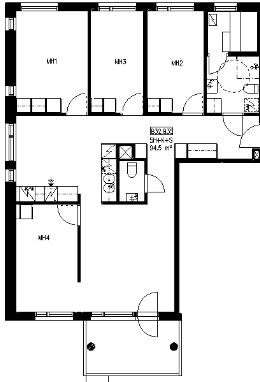
Särkilahdenkatu 1 B 32 / pohjakuva Ei mittakaavassa
