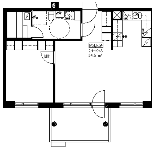
Särkilahdenkatu 1 B 34 / pohjakuva Ei mittakaavassa
