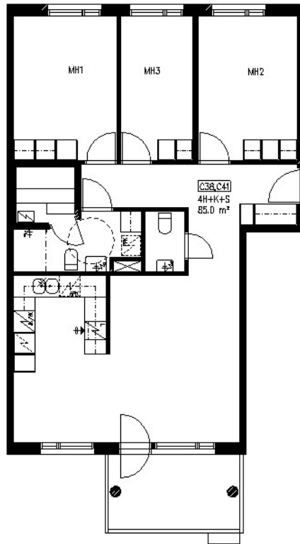
Särkilahdenkatu 1 C 41 / pohjakuva Ei mittakaavassa
