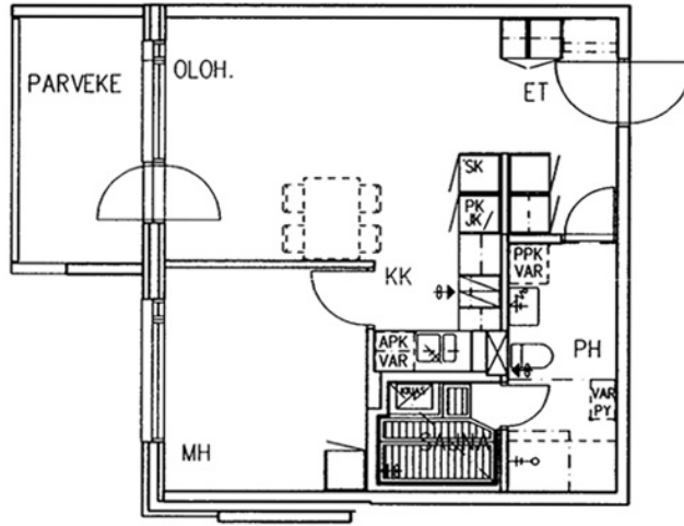
Sarvikatu 6 B 20 / pohjakuva Not in scale
