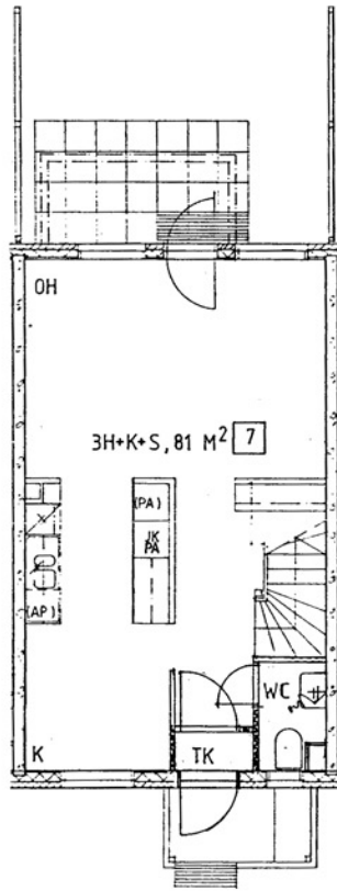
Kaskitie 14 B 7 / pohjakuva 1. kerros Ei mittakaavassa
