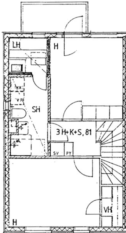
Kaskitie 14 B 10 / pohjakuva 2. kerros Ei mittakaavassa
