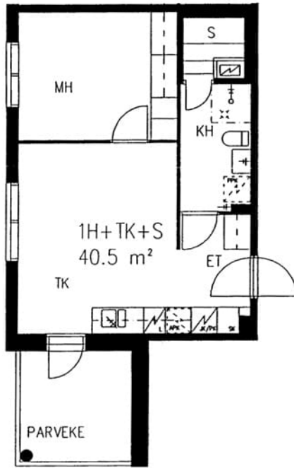
Lintulammenkatu 5 C A 16 / pohjakuva
