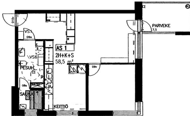
Hauenkouku 4 A 1 / pohjakuva Ei mittakaavassa
