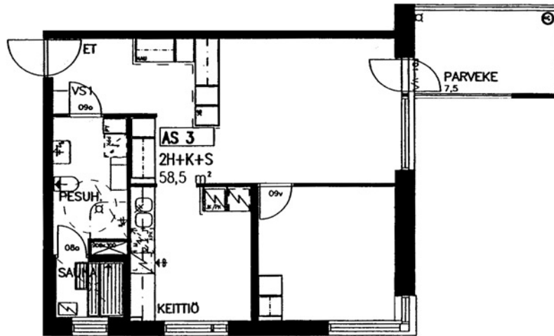
Hauenkouku 4 A 3 / pohjakuva Not in scale
