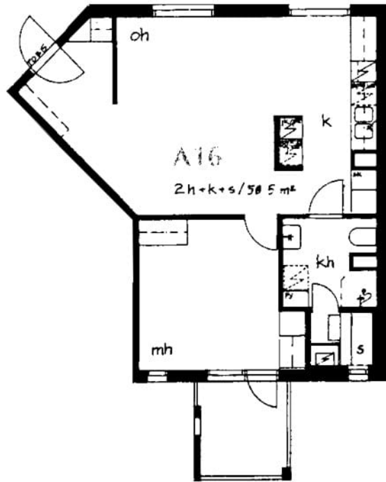
Kyyhkysmäki 12 A 16 / pohjakuva Not in scale
