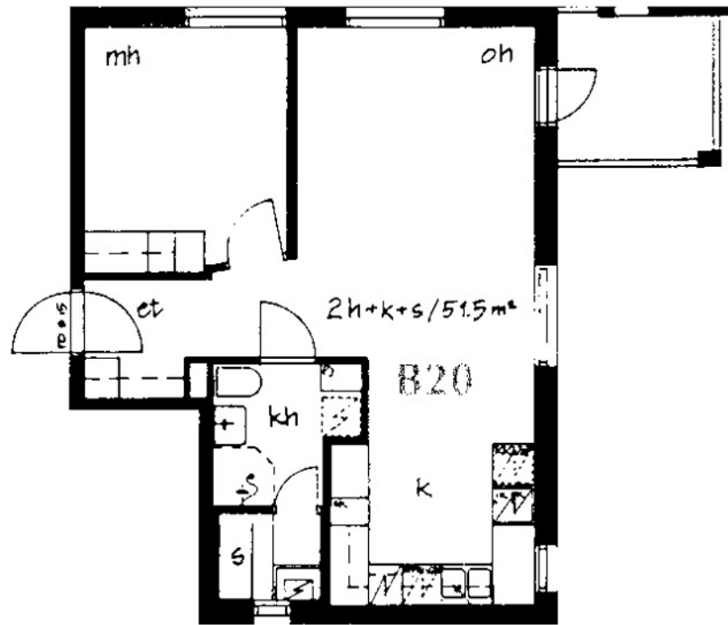
Kyyhkysmäki 12 B 20 / pohjakuva Ei mittakaavassa
