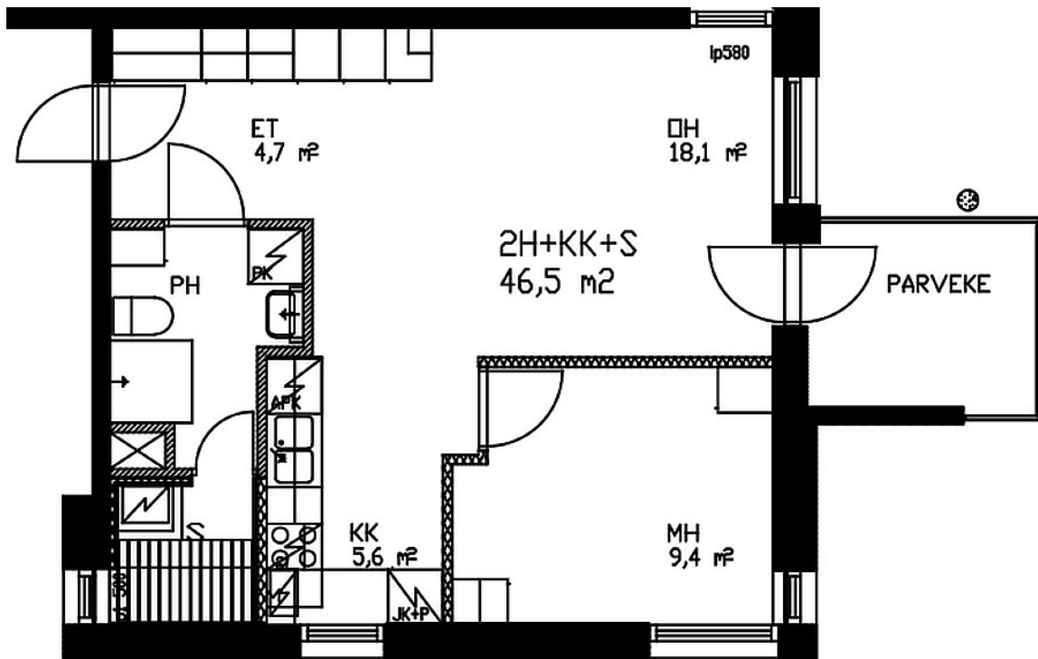
Tervaraitti 4 C 31 / Pohjakuva Ei mittakaavassa
