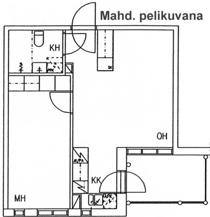
Kuusikonkatu 9 A 2 / pohjakuva Ei mittakaavassa
