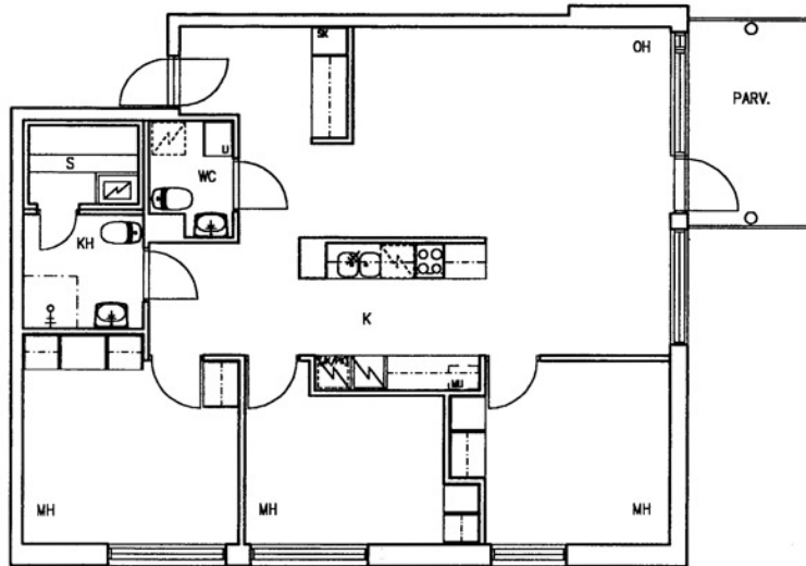
Tilanhoitajankaari 7 B 37 / pohjakuva Ei mittakaavassa
