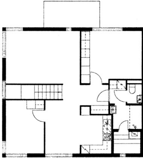
Sissosentie 20 E 19 / pohjakuva Ei mittakaavassa
