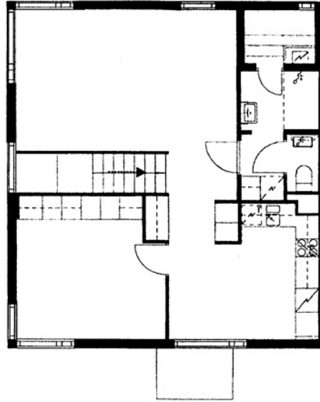
Sissosentie 15 A 2 / pohjakuva Ei mittakaavassa
