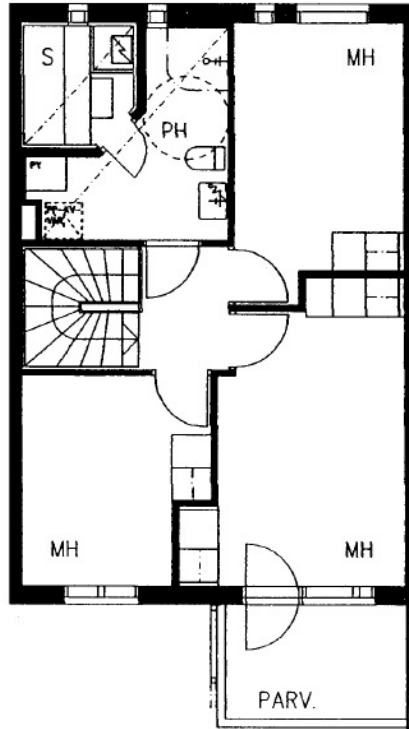
Kaivantokuja 2 A 3 / pohjakuva 2. kerros Ei mittakaavassa
