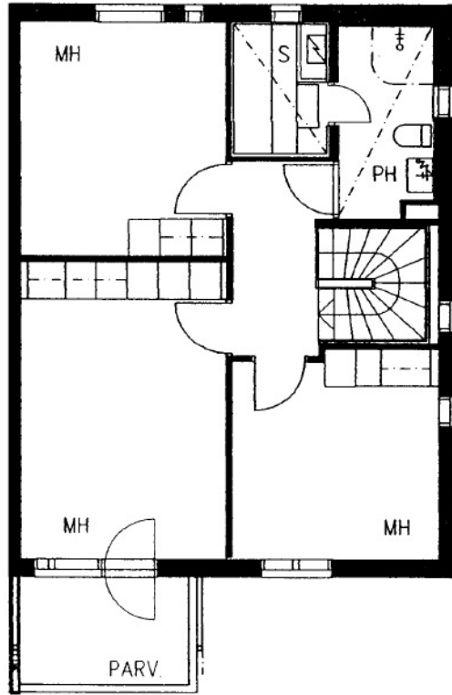
Kaivantokuja 2 C 14 / pohjakuva 2. kerros Not in scale
