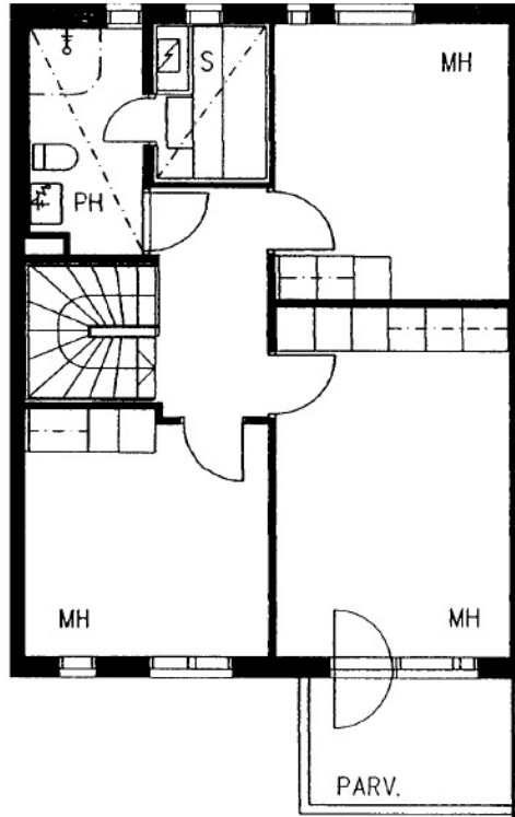
Kaivantokuja 2 C 15 / pohjakuva 2. kerros Ei mittakaavassa
