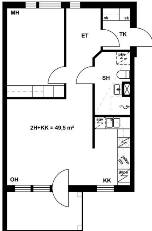
Ramsinniementie 7 A 3 / Pohjakuva Ei mittakaavassa
