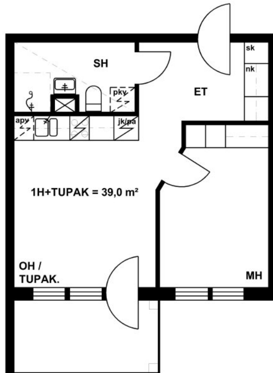
Ramsinniementie 7 L 82 / Pohjakuva Ei mittakaavassa
