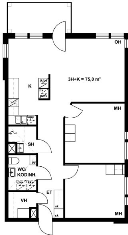
Ramsinniementie 7 K 79 / Pohjakuva Ei mittakaavassa
