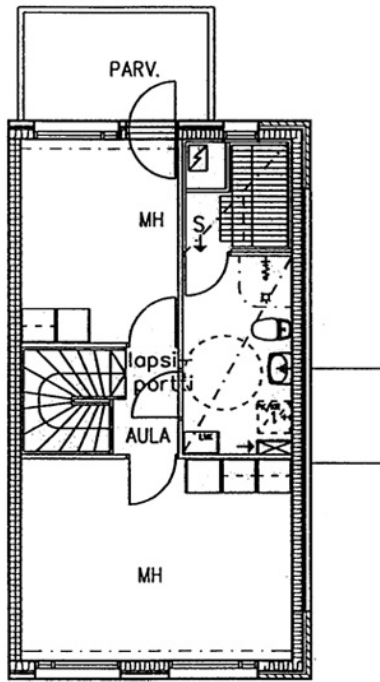
Liivurentie 11 E 15 / pohjakuva 2.kerros Ei mittakaavassa
