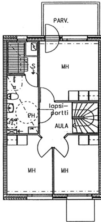
Liivurentie 11 C 8 / pohjakuva 2.kerros Ei mittakaavassa
