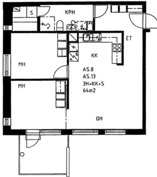
Asemakatu 4 A 8 / pohjakuva Ei mittakaavassa
